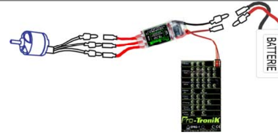
Schéma de branchement pour la programmation d'un contrôleur PROTRONIK
